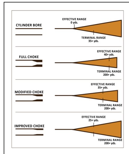
رسم 12 – المخنق المختلفة وتأثيراتها
